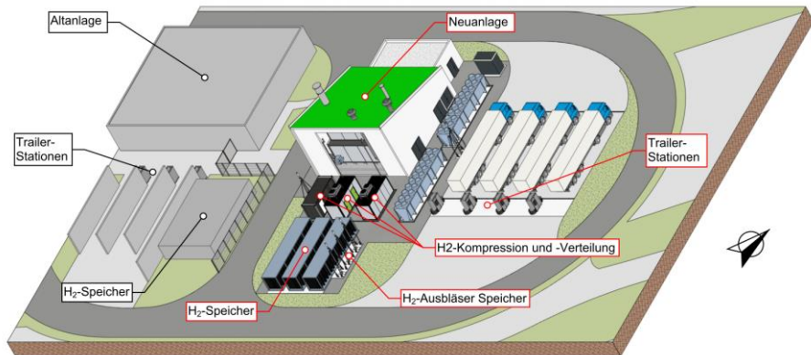
Abb. 2: Übersicht über das Vorhaben und die bestehende Anlage (Plant Engineering; Planstand: 22.12.2022)
